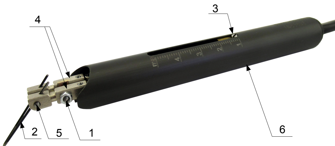
Рис. 1. Инструмент с установленным сдвоенным электродом.
